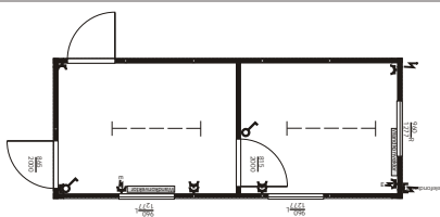
Raumcontainer mit Trennwand Ideal zur Nutzung als Ausstellungsraum mit separatem Büro-/Besprechungsraum
