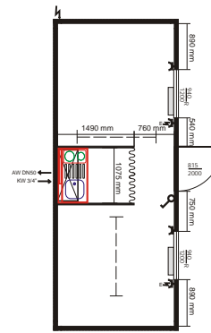
Raumcontainer mit zwei separaten Ausstellungsräumen inklusive abgetrennter Kleinküche!
